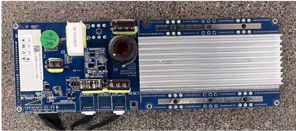
Photo 4 电池组保护板背面 Back view of PCM
