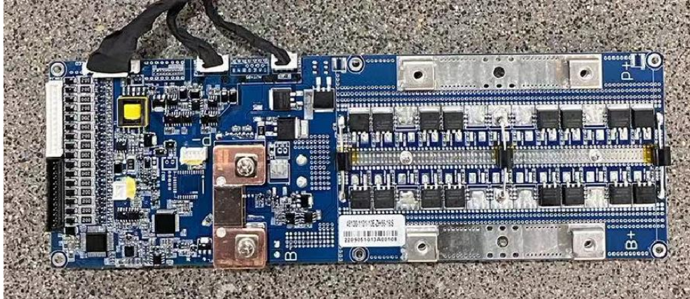
Photo 3 电池组保护板正面 Front view of PCM
